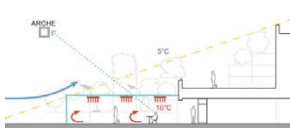
Schémas confort thermique Hiver
