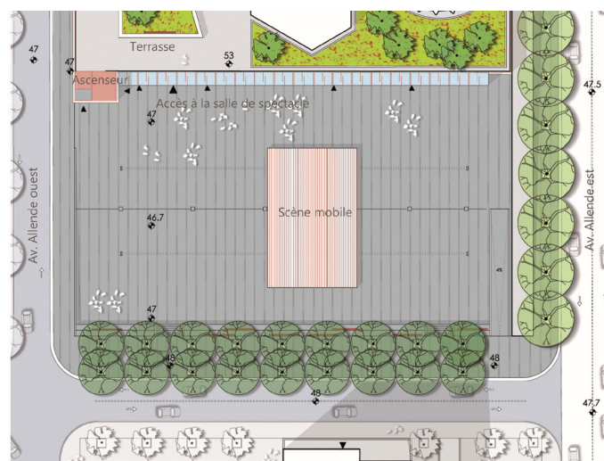
Aménagement de la place Rabin/Arafat
